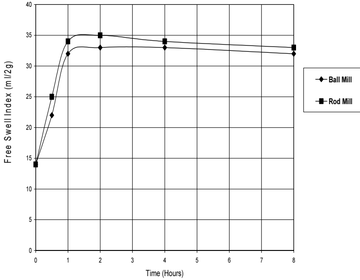
شكل رقم (٦). دليل الانتفاخ الحر للطحن الناعم لبيتونايت خليص مع ٦٪ كربونات صوديوم باستخدام طاحونة الكور والقضبان الصغيرة.
