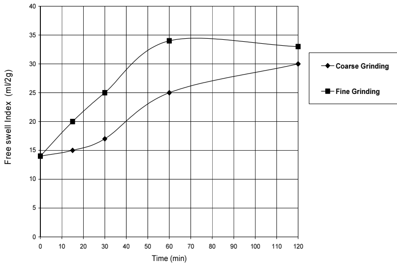
شكل رقم (٧). دليل الانتفاخ الحر للطحن الناعم والخشن لبيتونايت خليص مع ٦٪ كربونات صوديوم باستخدام الطحن اليدوي.
