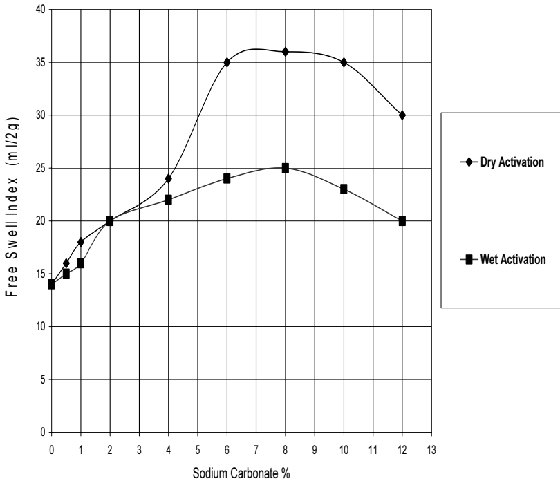
شكل رقم (٤). التنشيط الجاف والرطب عند نسب مختلفة لكربونات الصوديوم (بنتونايت خليص الناعم).
